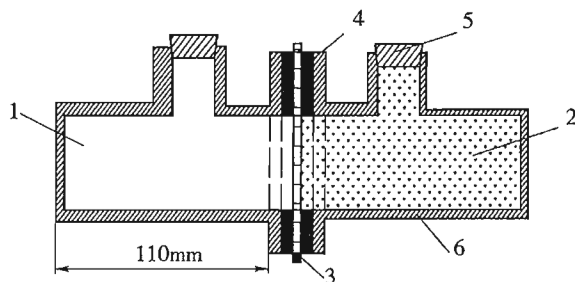
图 B.1 涂层抗氯离子渗透性试验装置示意图 1-3% NaCl 水溶液; 2-蒸馏水; 3-试件(活动涂层片); 4-硅橡胶填料; 5-硅橡胶塞; 6-内径为 40mm ~ 50mm 试验槽
